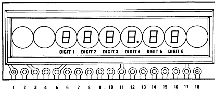
NSA1188*
